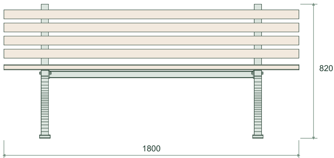
Вид спереди
